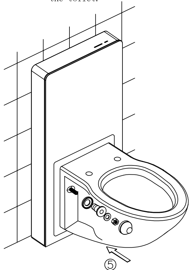
安装马桶 install toilet
