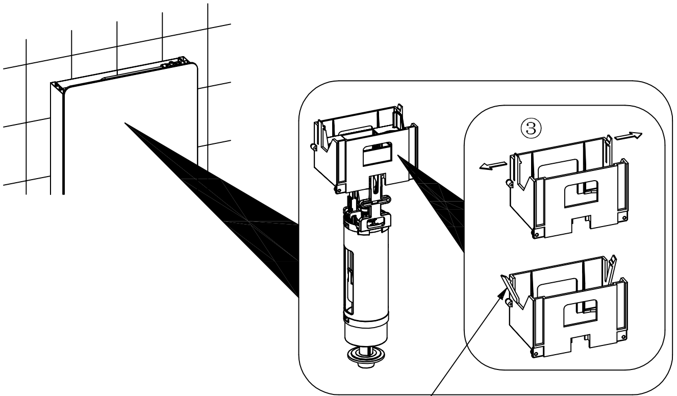
水箱挂板上的卡扣 buckles on the cistern hunger
