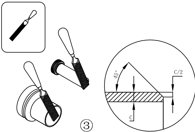
冲水直管和排水直管口部倒角
