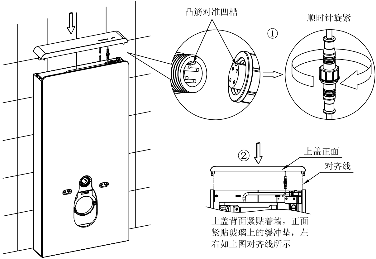
把上盖安装到柜体上
