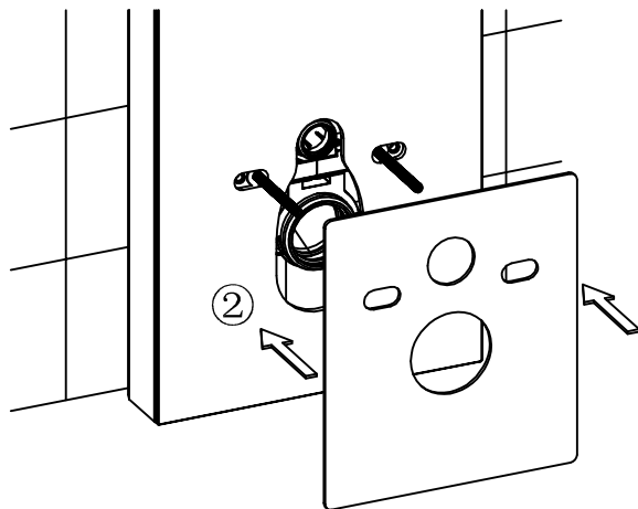
安装马桶缓冲垫 install toilet mat
