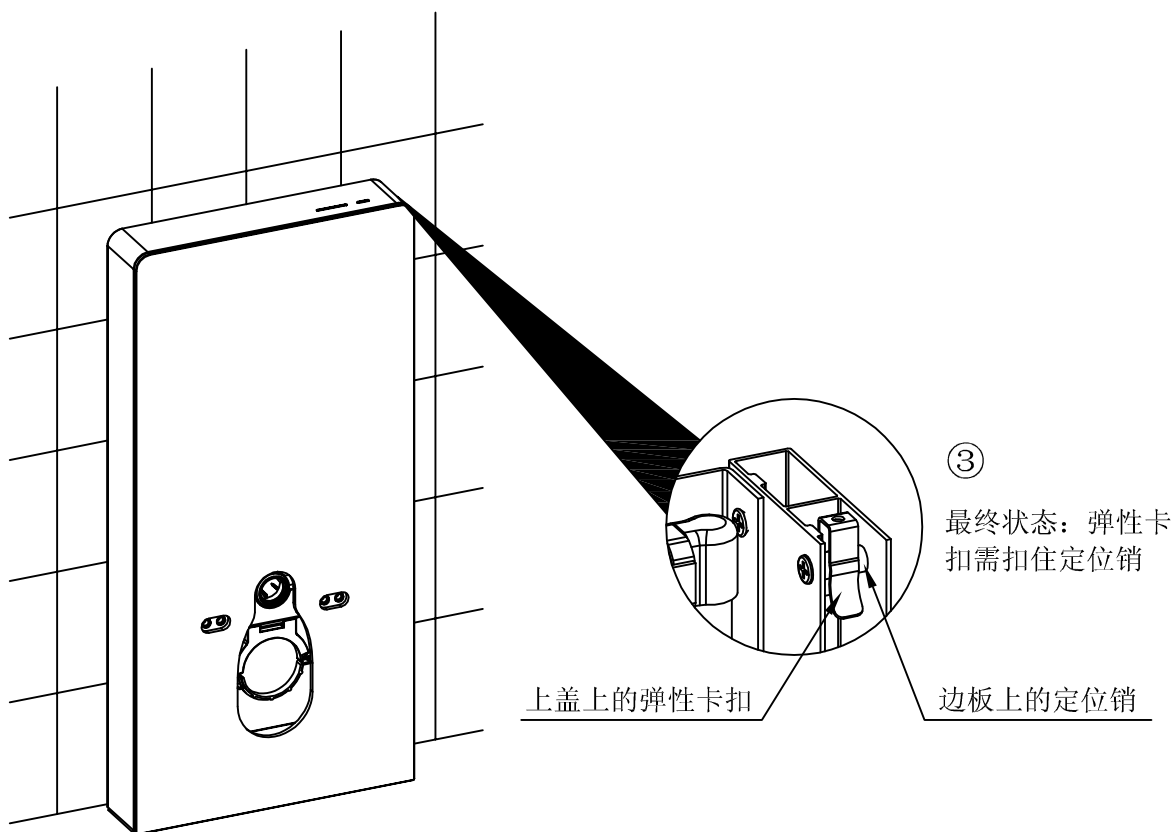
把上盖安装到柜体上
