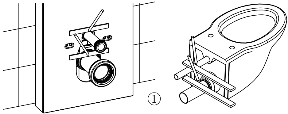
在冲水直管和排水直管上划线
